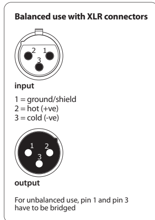
Fig. 3.1: Connettori XLR
