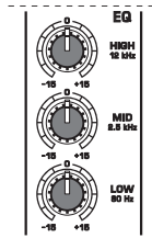
Fig. 2.5: Regolazione del suono dei canali di ingresso stereo
