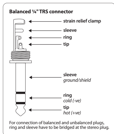
Fig. 3.3: Presa jack stereo 6,3 mm
