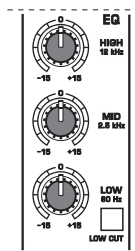
Fig. 2.2: regolazione del suono dei canali d'ingresso mono
