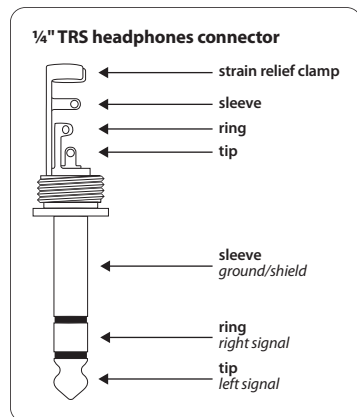
Fig. 3.4: Presa jack stereo per cuffia
