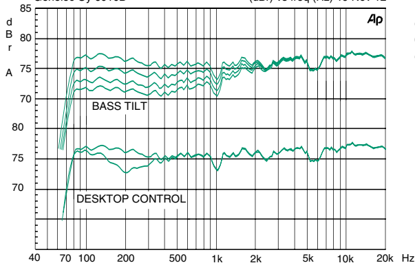
Kuva 4. Taajuusvast-esäätimien vaikutus 6010B:n toistovast-eeseen.
