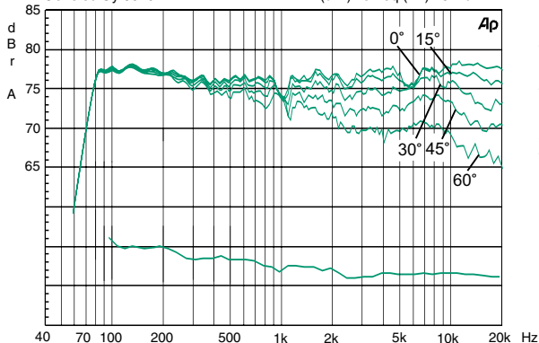
Kuva 5. Ylemmät käyrät esittävät 6010B:n taajuusvasteen eri kulmista mitattuna (kaiutin pystyasennossa, mittausetäisyys 1 m). Alempi käyrä on kaiuttimen tehovaste.
