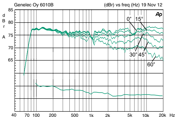
Abbildung 5. Die obere Kurvenschar zeigt die horizontale Abstrahlcharakteristik des 6010B gemessen in einem Meter Abstand. Die untere Kurve zeigt das Bündelungsmaß.
