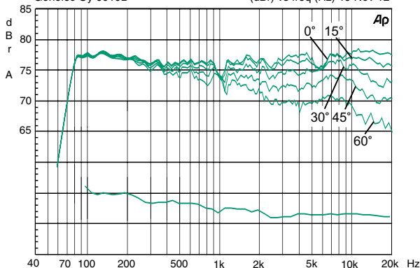
Illustration 5. Le groupe de courbes montre les caractéristiques de directivité horizontale de la 6010B mesurées à 1 m. La courbe inférieure montre la réponse en puissance de l'enceinte.
