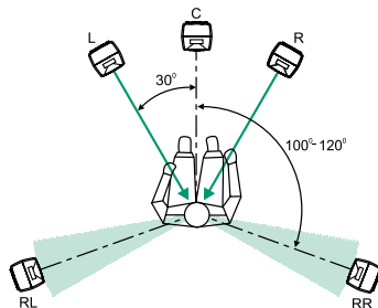
Kuva 2. Oikea kaiuttimien sijoittelu viisikanaisessa surround-järjestelmässä.
