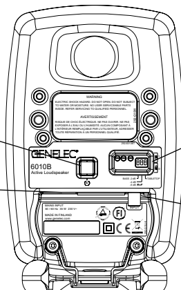
Figur 3: Kontrollernas och anslutningarnas placering på 6010B:s baksidespanel.
