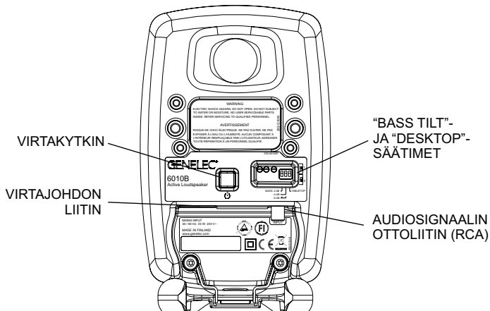
Kuva 3. 6010B:n liitännät ja säätimet.
