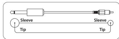
Fig. 5.2: cavo adattatore mono
