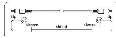
Fig. 5.1: cablaggio di un cavo cinch
