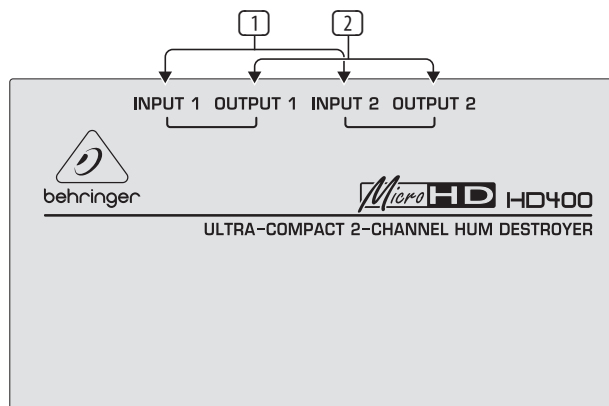
Collegamenti del HD400
