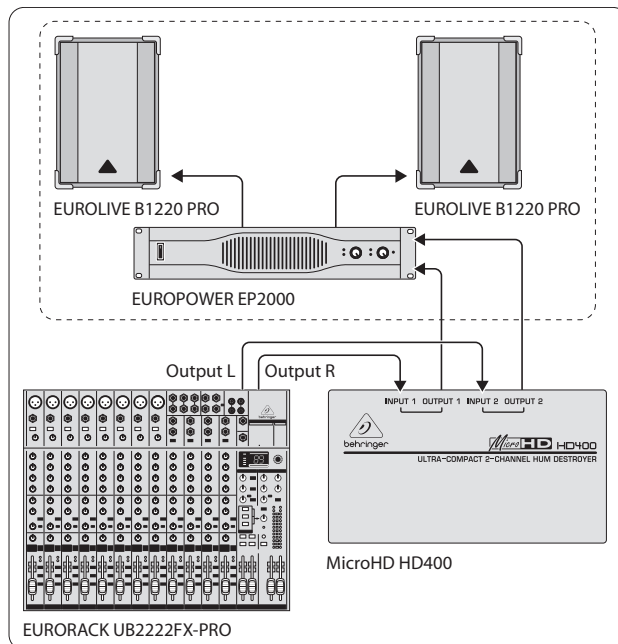
Cablaggio del HD400
